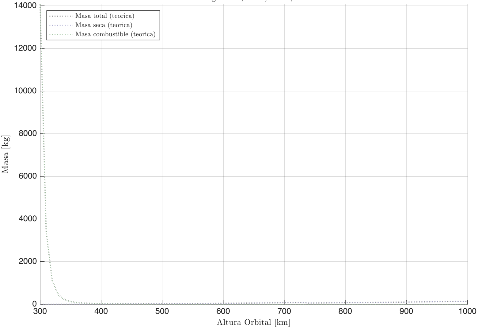
Desglose de Masas vs. Altura Config: 3 Sat, 1 Tel, Det 2, TMA
